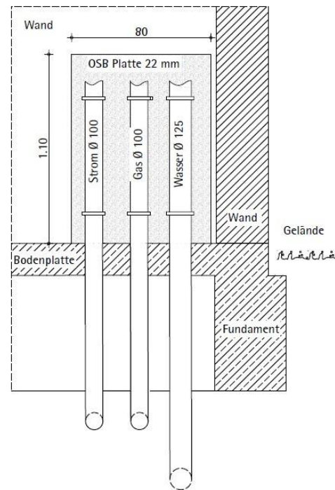
Ansicht Wand OSB Platte Hauseinführungen
