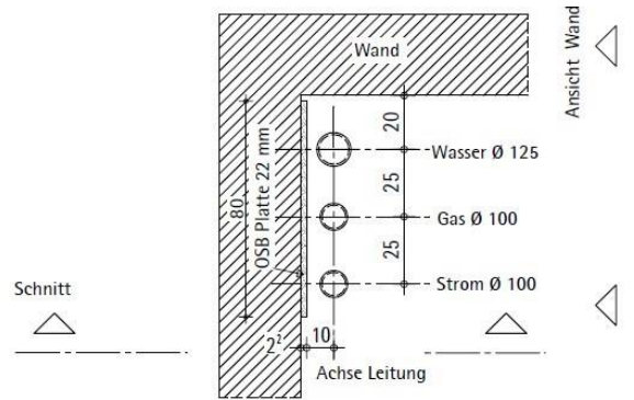
Grundriss Hauseinführungen
